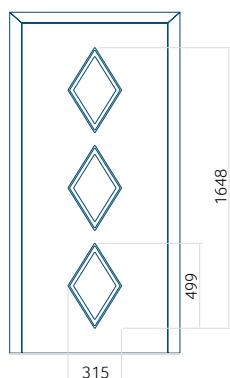
Dessin technique
