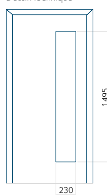
Dessin technique
